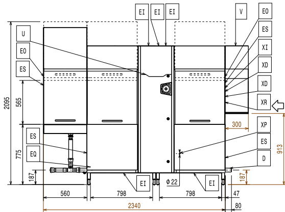
Zij aanzicht
